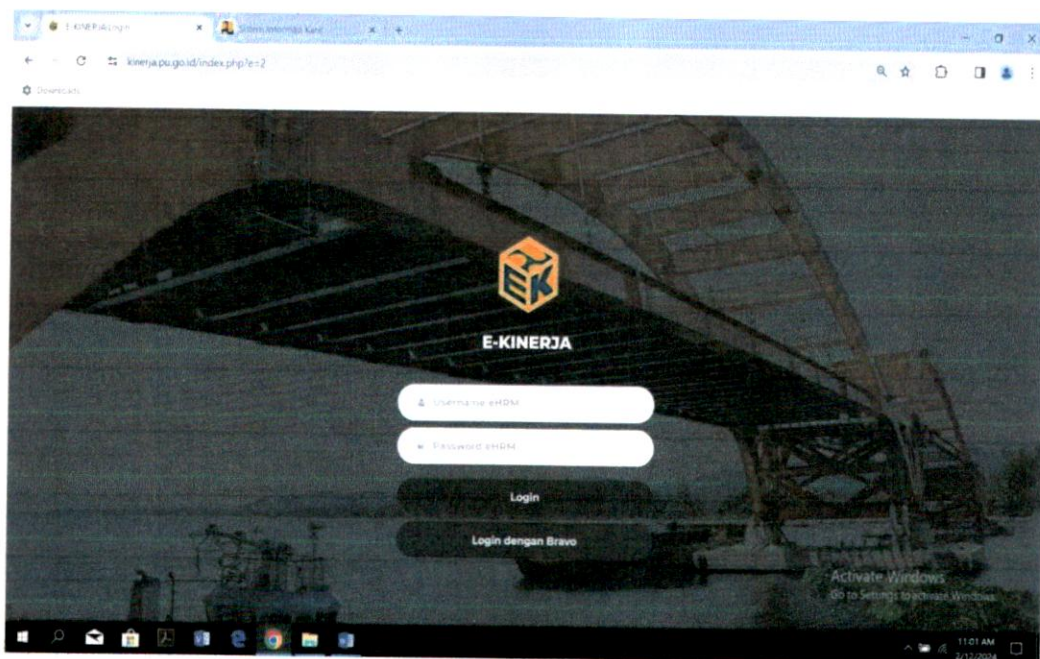
Gambar 1. Aplikasi E-Kinerja
