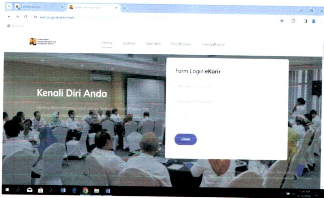
Gambar 2. Aplikasi E-Karir
